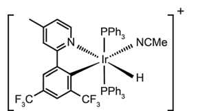
Ir[(CF 3 ) 2 Meppy](PPh 3 ) 2 (H)(NCMe) + 46
