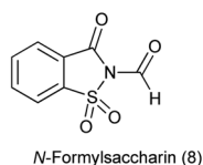
N -Formylsaccharin (8)
