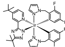
Ir(dfb-pz) 2 (bbptz)
