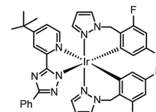
Ir(dfb-pz) 2 (pbptz)
