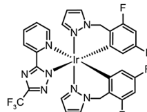
Ir(dfb-pz) 2 (fptz)
