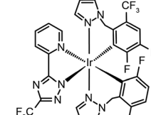
Ir(tfmb-pz) 2 (fptz)
