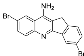
3,8-Dibromo-11H-indeno[1,2-b]quinolin-10-amine
