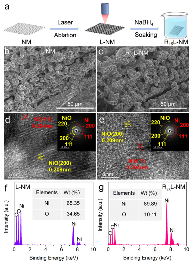
Fig. 1 (a) Schematic illustration of R 15 L-NM. (b) and (c) SEM images of L-NM and R 15 L-NM. (d) and (e) STEM-EDX mapping of L-NM and R 15 L-NM. (f) and (g) EDX spectra of L-NM and R 15 L-NM.
