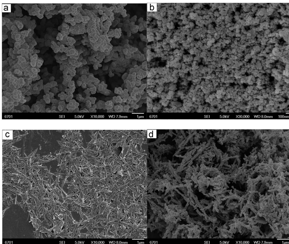
Fig. 2 SEM micrographs of PPy (a), \text{Fe}_3\text{O}_4 (b), ATP (c) and \text{PPy}/\text{Fe}_3\text{O}_4/\text{ATP} (d) composite.
