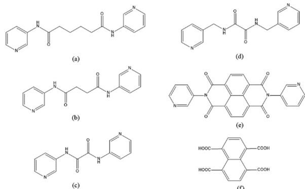
Fig. 1 Structures of (a) L 1 , (b) L 2 , (c) L 3 , (d) L 4 , (e) L 5 and (f) 1,4,5,8-H 4 NTC.
