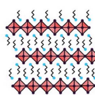
A-site
