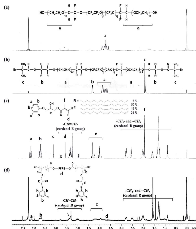
Fig. 2 1 H NMR spectrum of (a) E10H, (b) Br–PFPE–Br, (c) HCPM, and (d) PHCPMF30.
