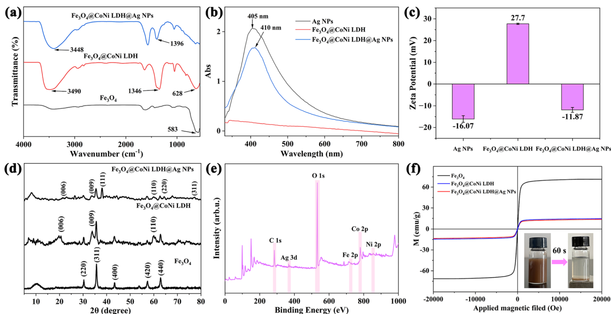
Fig. 2 (a) FT-IR spectra of \text{Fe}_3\text{O}_4 , \text{Fe}_3\text{O}_4@\text{CoNi LDH} and \text{Fe}_3\text{O}_4@\text{CoNi LDH}@\text{Ag NPs} ; (b) UV-visible absorption spectra of Ag NPs, \text{Fe}_3\text{O}_4@\text{CoNi LDH} and \text{Fe}_3\text{O}_4@\text{CoNi LDH}@\text{Ag NPs} ; (c) zeta potentials of Ag NPs, \text{Fe}_3\text{O}_4@\text{CoNi LDH} , and \text{Fe}_3\text{O}_4@\text{CoNi LDH}@\text{Ag NPs} ; (d) XRD patterns of \text{Fe}_3\text{O}_4 , \text{Fe}_3\text{O}_4@\text{CoNi LDH} and \text{Fe}_3\text{O}_4@\text{CoNi LDH}@\text{Ag NPs} ; (e) XPS survey of \text{Fe}_3\text{O}_4@\text{CoNi LDH}@\text{Ag NPs} ; and (f) magnetic hysteresis loops.
