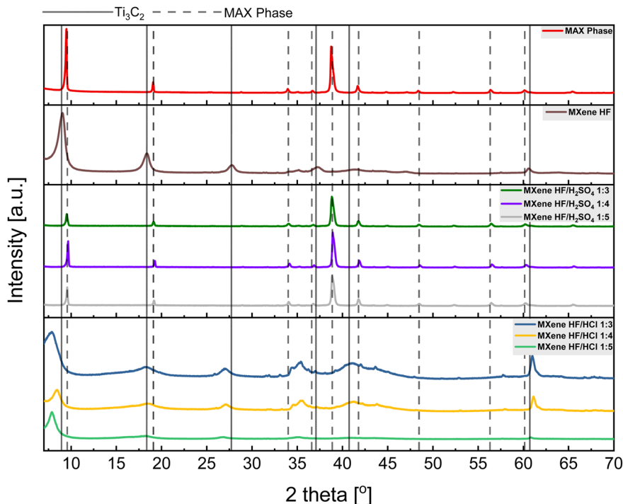
Fig. 2 XRD patterns of MAX phase, MXene HF, MXenes HF/ \text{H}_2\text{SO}_4 1 : 3, 1 : 4, 1 : 5 and MXenes HF/HCl 1 : 3, 1 : 4, 1 : 5.
