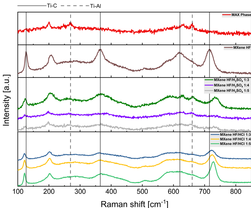
Fig. 3 Raman spectra of MAX phase, MXene HF, MXenes HF/ \text{H}_2\text{SO}_4 1 : 3, 1 : 4, 1 : 5 and MXenes HF/HCl 1 : 3, 1 : 4, 1 : 5.
