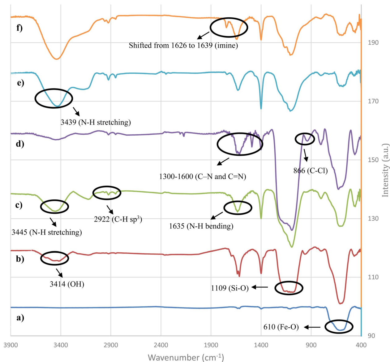
Fig. 1 FT-IR spectra of (a) \text{Fe}_3\text{O}_4 , (b) \text{SiO}_2 @ \text{Fe}_3\text{O}_4 , (c) APTES@ \text{SiO}_2 @ \text{Fe}_3\text{O}_4 , (d) TCT/APTES@ \text{SiO}_2 @ \text{Fe}_3\text{O}_4 , (e) picolylamine/TCT/APTES@ \text{SiO}_2 @ \text{Fe}_3\text{O}_4 , and (f) \text{Ni}^{\text{II}} -picolylamine/TCT/APTES@ \text{SiO}_2 @ \text{Fe}_3\text{O}_4 .
