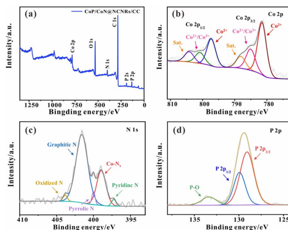
Fig. 3 (a) XPS spectrum, (b) Co 2p, (c) N 1s, and (d) P 2p of CoP/CoN@NCNRs/CC.
