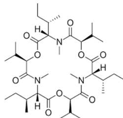
Enniatin B
