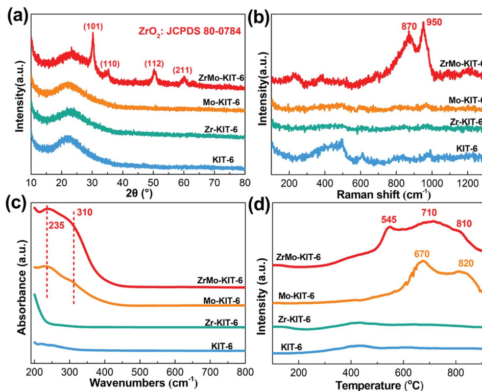
Fig. 2 (a) WAXRD patterns, (b) Raman spectra, (c) UV-vis spectra, and (d) H 2 -TPR patterns of KIT-6, Zr-KIT-6, Mo-KIT-6, and ZrMo-KIT-6.
