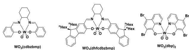
Fig. 33 Tungsten(VI) complexes.
