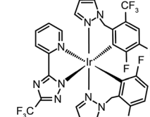
Ir(tfmfb-pz) 2 (fptz) 54
