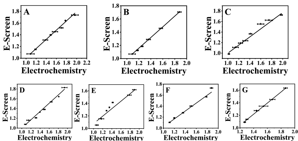
Fig. 4 Correlation fitting diagram between electrochemical method and E-Screen method. (A) GA 3 (B) ETH, (C) NAA, (D) GA 3 : ETH = 1 : 1, (E) GA 3 : NAA = 1 : 1, (F) ETH : NAA = 1 : 1, (G) GA 3 : ETH : NAA = 1 : 1 : 1.
