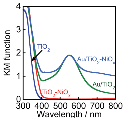
Fig. 2 Absorption spectra of TiO 2 , TiO 2 -NiO x (0.5), Au(1.0)/TiO 2 , and Au(1.0)/TiO 2 -NiO x (0.5).
