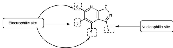
Fig. 18 Pyrazolo-pyridine.
