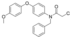
CCW16 (RNF4)
