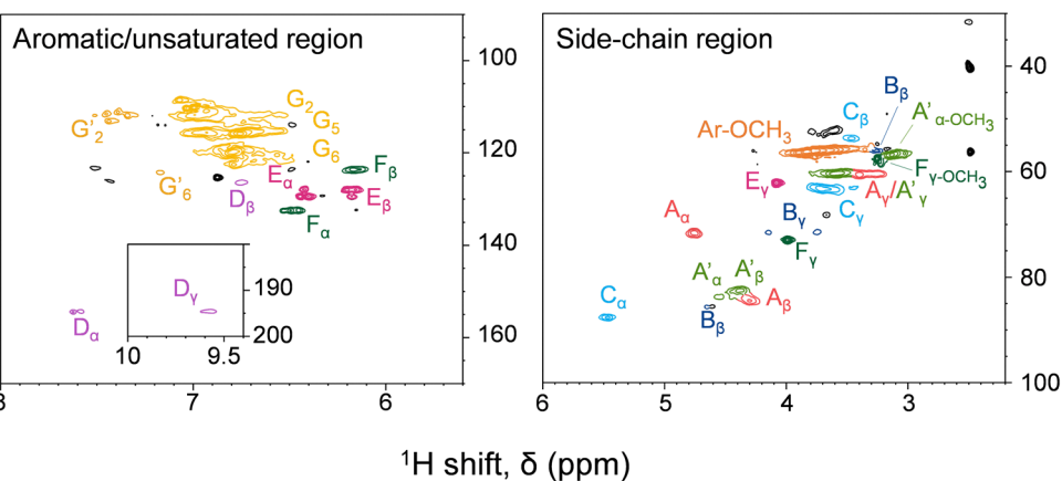
(b) 30 MPa
