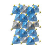
Cu 3 SnS 4 - kuramite
