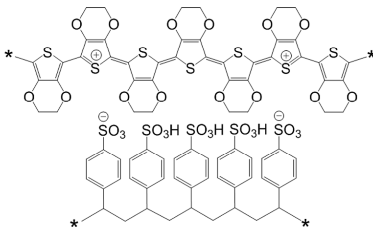
PEDOT:PSS
