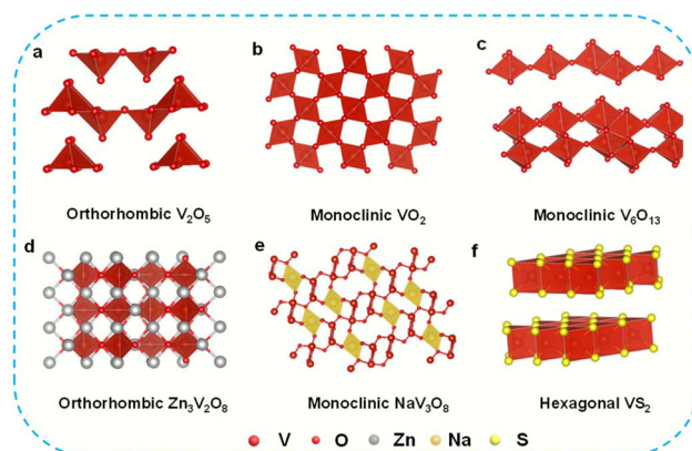
Fig. 2 Crystal structure of V 2 O 5 , VO 2 , V 6 O 13 , Zn 3 V 2 O 8 , NaV 3 O 8 , VS 2 .
