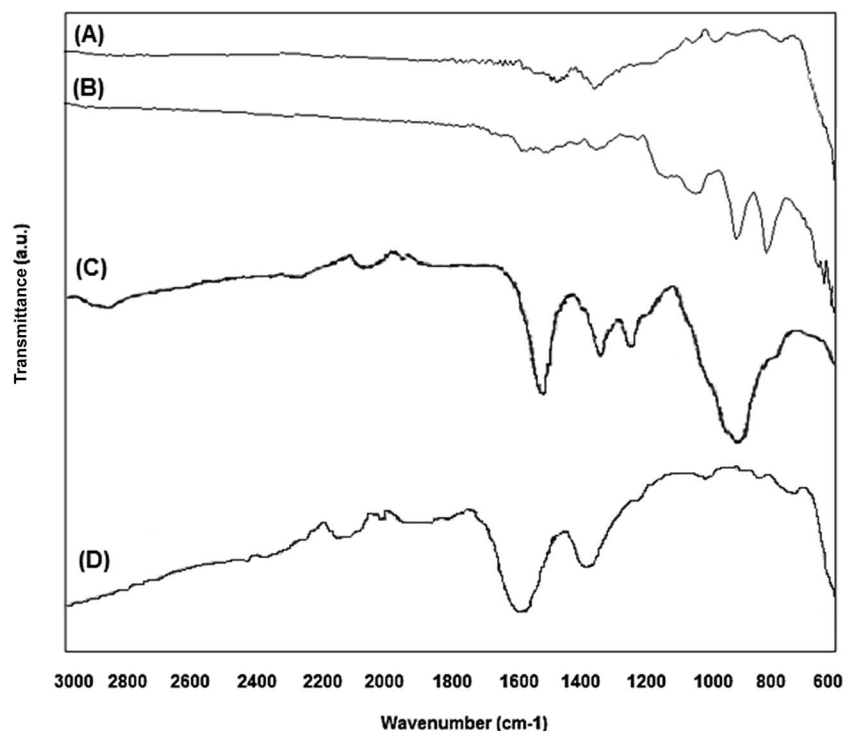
Fig. 3 Fourier transform infrared spectra of the prepared magnetic nanoparticles: (A) \text{Fe}_3\text{O}_4 ; (B) \text{Si}-\text{Fe}_3\text{O}_4 ; (C) pure CMC; (D) \text{Si}-\text{Fe}_3\text{O}_4@\text{CMC} .
