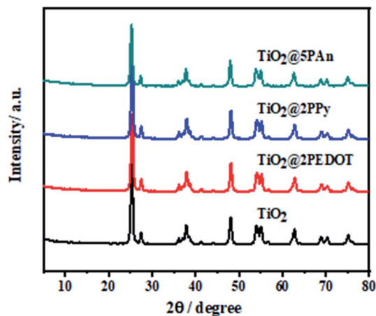
Fig. 4 X-ray diffraction patterns of TiO 2 , TiO 2 @2PEDOT, TiO 2 @2PPy, and TiO 2 @5PAn.
