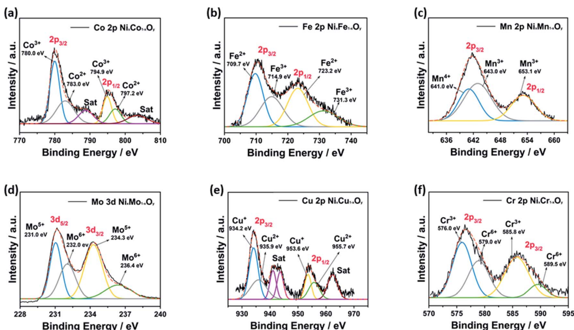
Fig. 6 XPS analysis of (a) Co 2p of Ni x Co 1-x O y , (b) Fe 2p of Ni x Fe 1-x O y , (c) Mn 2p of Ni x Mn 1-x O y , (d) Mo 3d of Ni x Mo 1-x O y , (e) Cu 2p of Ni x Cu 1-x O y , (f) Cr 2p of Ni x Cr 1-x O y .
