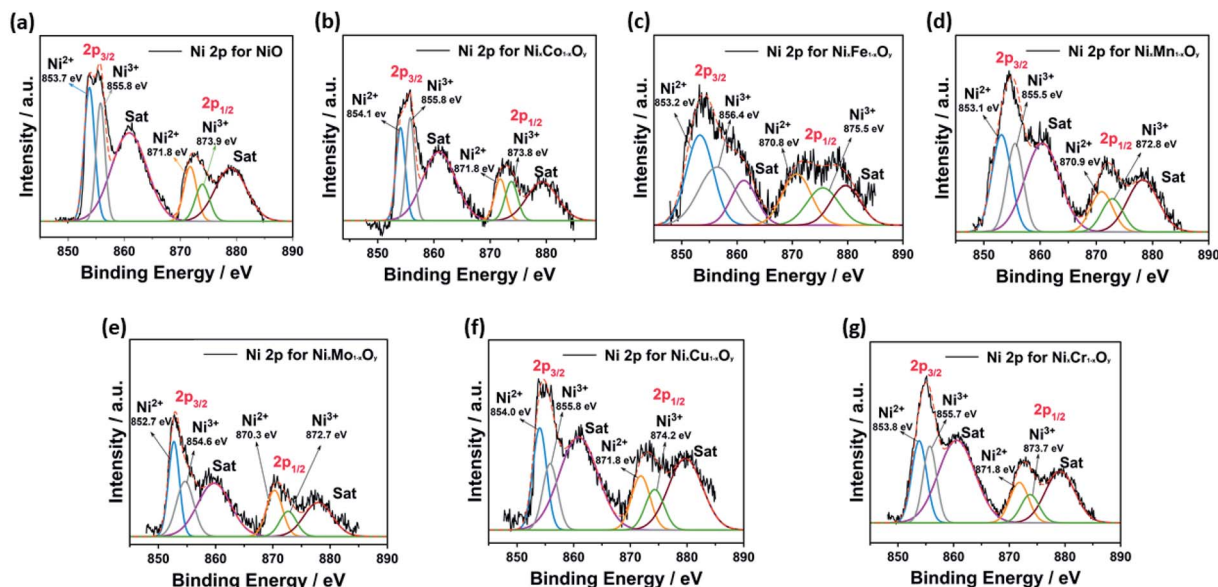
Fig. 5 Ni 2p spectrum for (a) NiO, (b) Ni x Co 1-x O y , (c) Ni x Fe 1-x O y , (d) Ni x Mn 1-x O y , (e) Ni x Mo 1-x O y , (f) Ni x Cu 1-x O y and (g) Ni x Cr 1-x O y .
