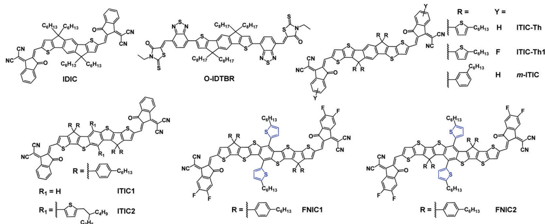
Fig. 27 Side-chain engineering of FREAAs.
