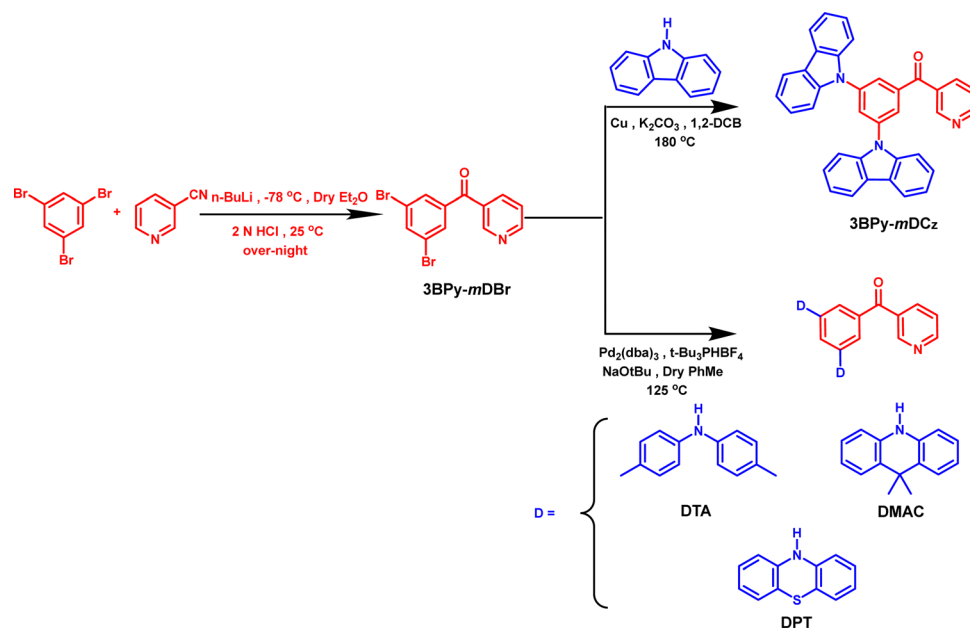
Scheme 1 Synthesis of 3BPpy-mDCz , 3BPpy-mDTA , 3BPpy-mDMAC and 3BPpy-mDPT .
