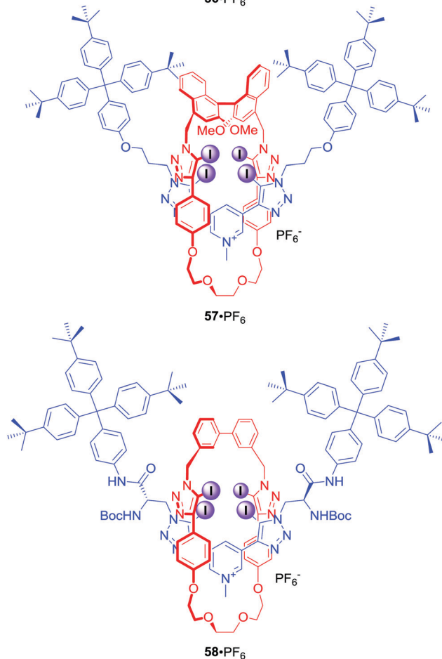
Fig. 26 Chiral XB [3]rotaxanes.
