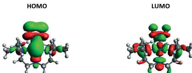
(c) [Pd(Bu 4 dien)(NO 2 )] + (reference 38)
