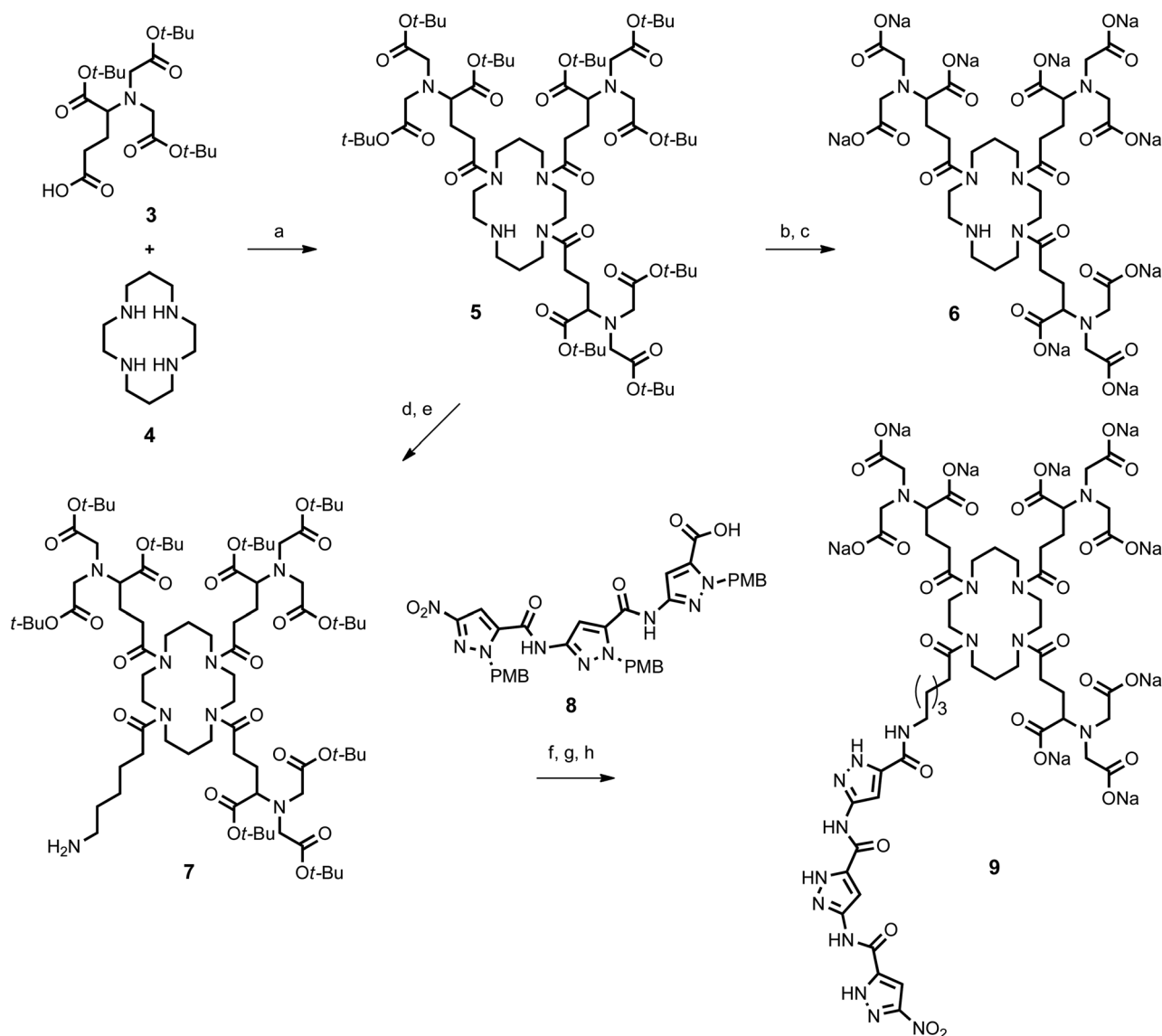
Fig. 5 Synthesis of cyclam-tris(NTA) sodium salt (6) and aminopyrazol-trimer-cyclam-tris(NTA) sodium salt (9). (a) TBTU, DIEA, CH 2 Cl 2 , rt, 24 h, 46%; (b) CH 2 Cl 2 /TFA 7:1, rt, 24 h, 88%; (c) 1 M NaOH, rt, 10 min, 99%; (d) Cbz-6-aminohexanoic acid, TBTU, DIEA, CH 2 Cl 2 , rt, 24 h, 85%; (e) H 2 , Pd/C, MeOH, 90%; (f) HCTU, Cl-HOBt, DIEA, CH 2 Cl 2 /DMF 2:1, 0 °C→rt, 48 h, 33%; (g) TFA, 70 °C, 5 h, 85%; (h) NaOH, Et 2 O, MeOH, 75%.
