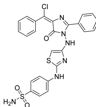
4-((4-((4-(Chlorobenzylidene)-5-oxo-2-phenyl-4,5-dihydro-1H-imidazol-1-yl)amino)thiazol-2-yl)amino)benzenesulfonamide
