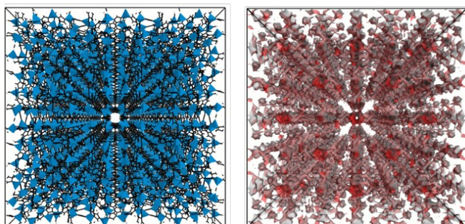
a_g ZIF-4
