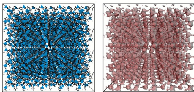
ZIF-zni
