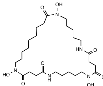
73, desferrioxamine E
