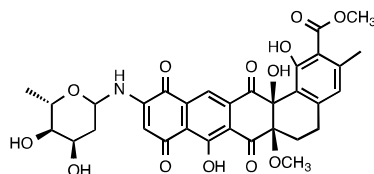
43, arenimycin A
