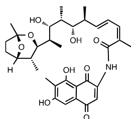
42, salinisporamycin
