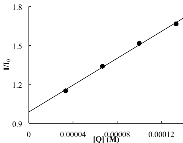
Fig. 8. Stern-Volmer plot for aqueous Au heli-viologen.
