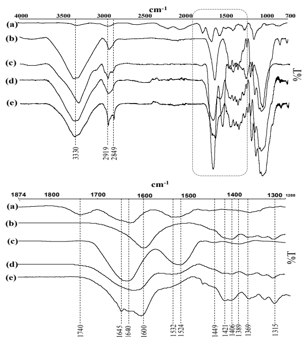
Figure 4. FT-IR spectra of the (a) Nisin, (b) CNF Tempo, (c) CNF Tempo-m-Nisin (d) CNF Tempo-g-1-eq and (e) CNF Tempo-g-4eq
