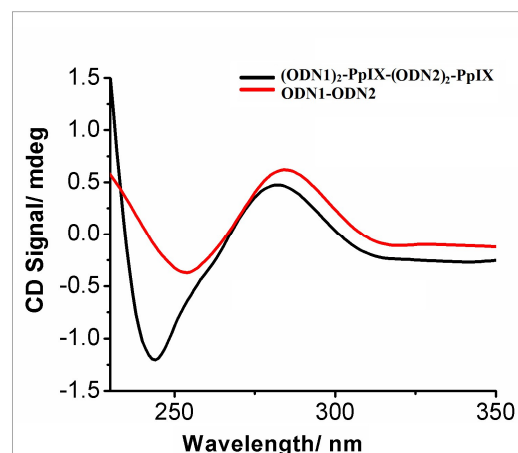
Fig.5 Circular dichroism of normal ODN1-ODN2 and (ODN1) 2 -PpIX - (ODN2) 2 -PpIX
