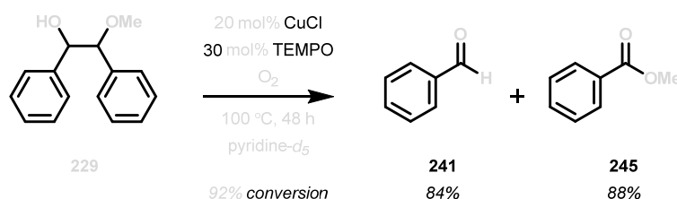
Scheme 22. Aerobic oxidation of 1,2-diphenyl-2-methoxyethanol ( 229 ).
