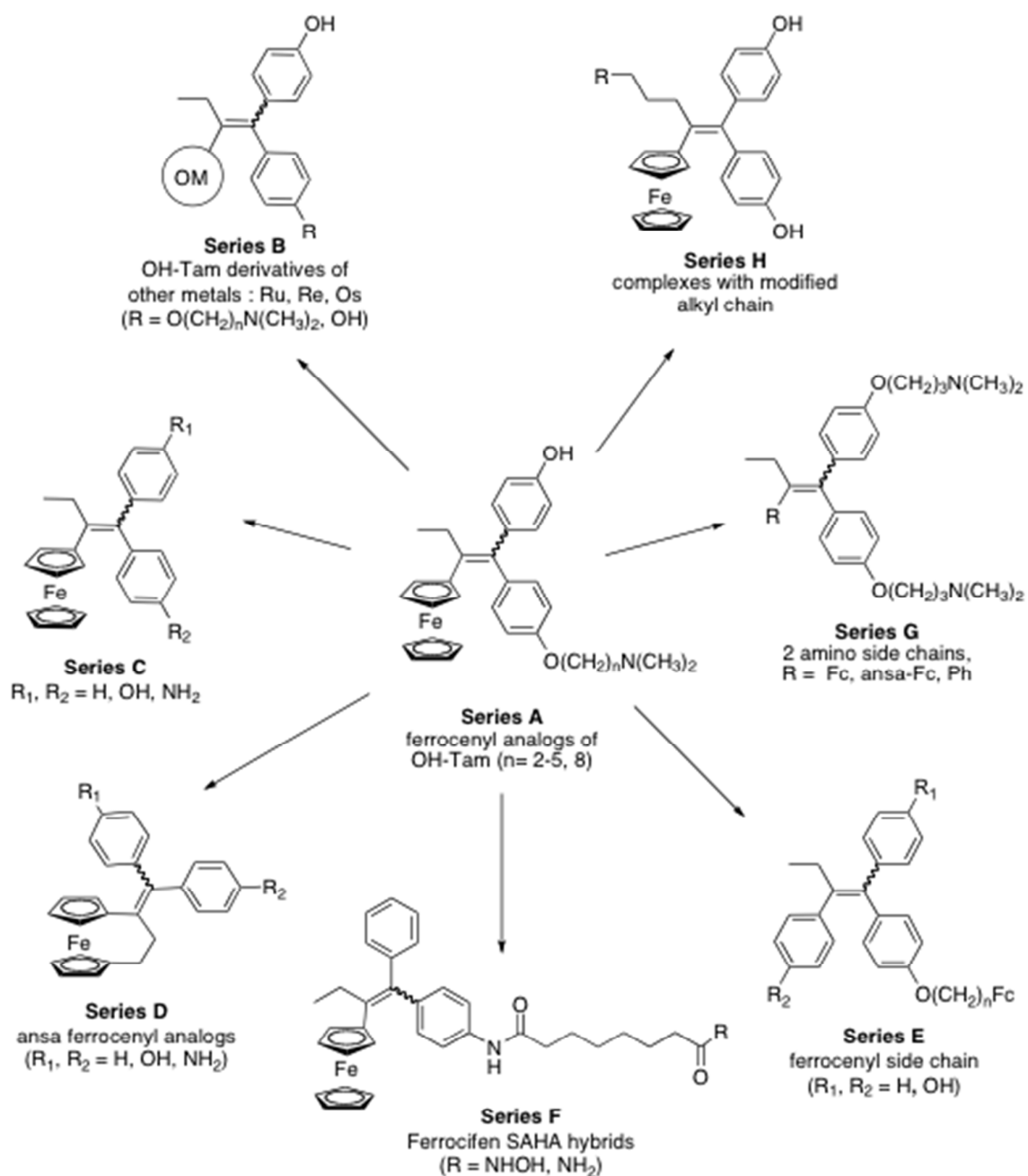
Chart 4 : Selected ferrocifens
