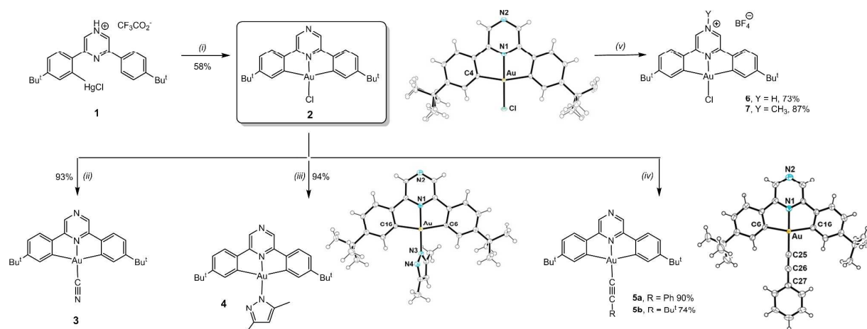
Scheme 1. Conditions: (i) KAuCl 4 , CH 3 CN/H 2 O 1:1, reflux 72h. (ii) KCN, CH 2 Cl 2 , 20 °C, 24 h. (iii) KO t Bu, 3,5-dimethylpyrazole, toluene, 20 °C, 6 h. (iv) AgC≡CR, CH 2 Cl 2 , 20 °C, 24 h. (v) HBF 4 ·Et 2 O, Et 2 O, 20 °C, 30 min. ( 6 ), or [Me 3 O]BF 4 , toluene/1,2-C 6 H 4 F 2 (5:1 v/v), 12 h. ( 7 ). Molecular structures [selected bond distances (Å) and angles (°)]: 2: Au-N1 1.976(4), Au-Cl 2.2653(12), Au-C4 2.078; N1-Au-C4 81.36(9), C4-Au-Cl 98.64(9), C4-Au-C4' 162.71(18), N1-Au-Cl 180. 4: Au-N1 1.979(2), Au-C6 2.080(3), Au-C16 2.073(3), Au-N3 1.991(2); C6-Au-N1 81.39(10), C16-Au-N1 81.32(11), C6-Au-N3 98.88(10), C16-Au-N3 98.38(11), N1-Au-N3 178.33(9). 5a: Au-N1 1.997(5), Au-C6 2.070(6), Au-C16 2.083(7), Au-C25 1.979(7), C25-C26 1.199(9); N1-Au-C6 80.4(2), N1-Au-C16 81.2(2), C6-Au-C25 99.3(3), C16-Au-C25 99.0(3), C6-Au-C16 161.6(3), Au-C25-C26 175.9(6), C25-C26-C27 177.4(7).
