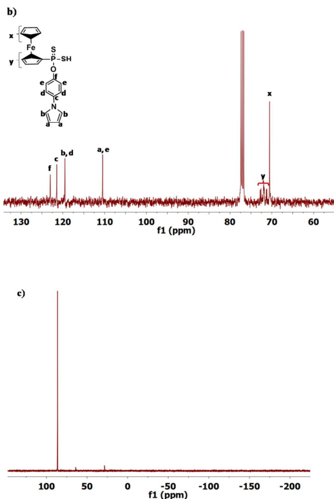
Fig. 1. a) ^1\text{H} -NMR, b) ^{13}\text{C} -NMR and c) ^{31}\text{P} -NMR spectra of the TpFc.
