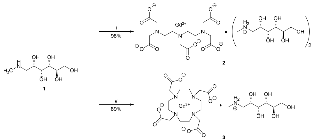
Scheme 1. Reactants and conditions: i = 1) DTPA, H 2 O, ))) , 2 min; 2) Gd 2 O 3 , H 2 O, ))) , 10 min; 3) another equiv of 1, ))) , 18 min. ii = 1) DOTA, H 2 O, ))) , 3 min; 2) Gd 2 O 3 , H 2 O, ))) , 17 min.
