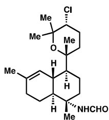
53: kalihinene E
