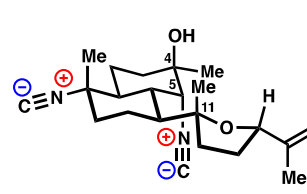
10: Kalihinol C
