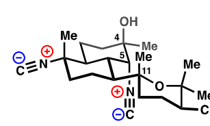
12: Kalihinol A
