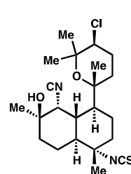
58: 10-epi-kalihinol X
