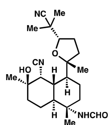
57: 10-formamido kalihinol F
