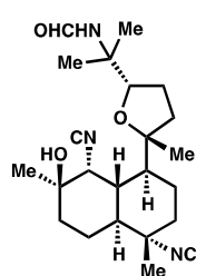
56: 15-formamido kalihinol F
