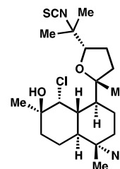
66: kalihinol T
