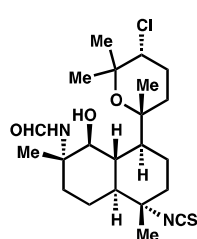
60: kalihinol N
