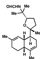
54: kalihinene F
