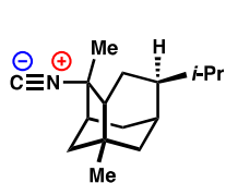
1: 2-Isocyanotrachyopsanes
