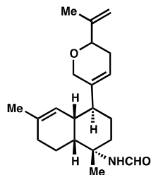
55: kalihipyran
