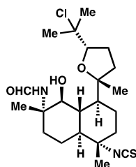
59: kalihinol M
