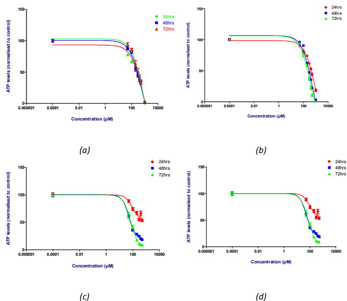
Fig. 3. Cell viability studies of triphenylarsonium derivatives 3 and 4 : (a), Cell Titre Glo assay of zwitterion 3 ; (b) Cell Titre Glo assay of thioacetate salt 4 ; (c), MTT assay of 3 ; (d) MTT assay of 4 .
