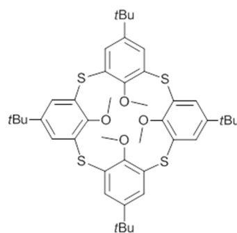
Fig. 1 p -tert-Butyltetramethoxythiacalix[4]arene 1
