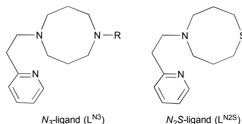
Fig. 1 Ligand structures.
