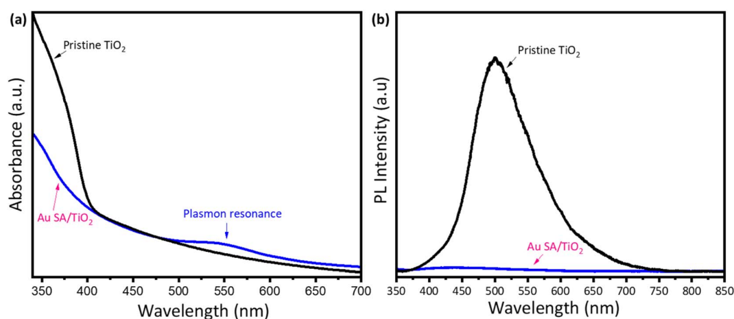
Fig. 5 The UV-vis absorption spectra of pristine TiO_2 and Au SA/ TiO_2 , respectively (a) and (b).
