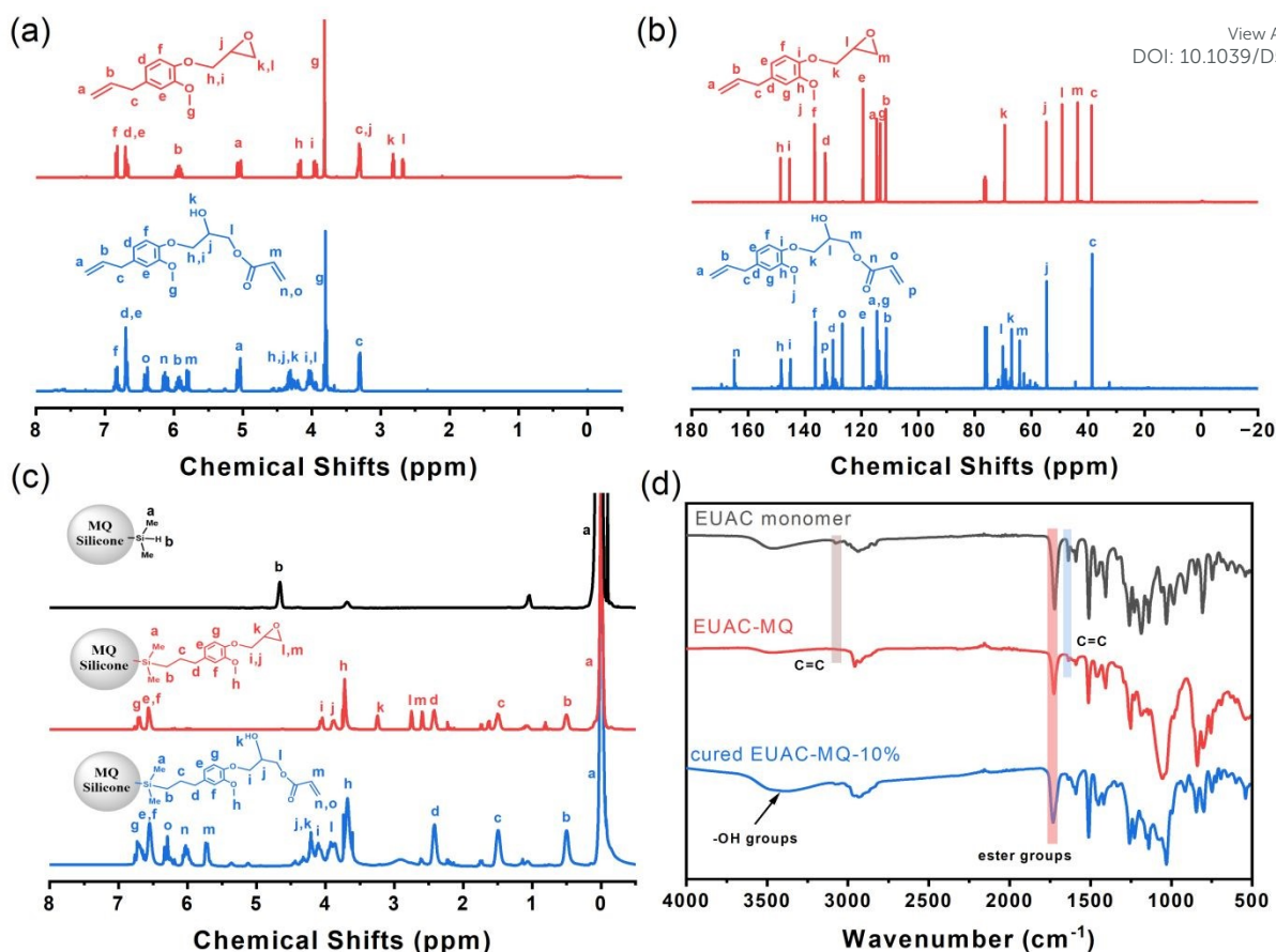
Fig. 3 NMR spectra of EUAC and EUAC-MQ (a) 1 H NMR; (b) 13 C NMR; (c) 1 H NMR spectrum of EUAC-MQ; (d) FT-IR spectra of EUAC, EUAC-MQ, and EUAC-MQ-10%.
